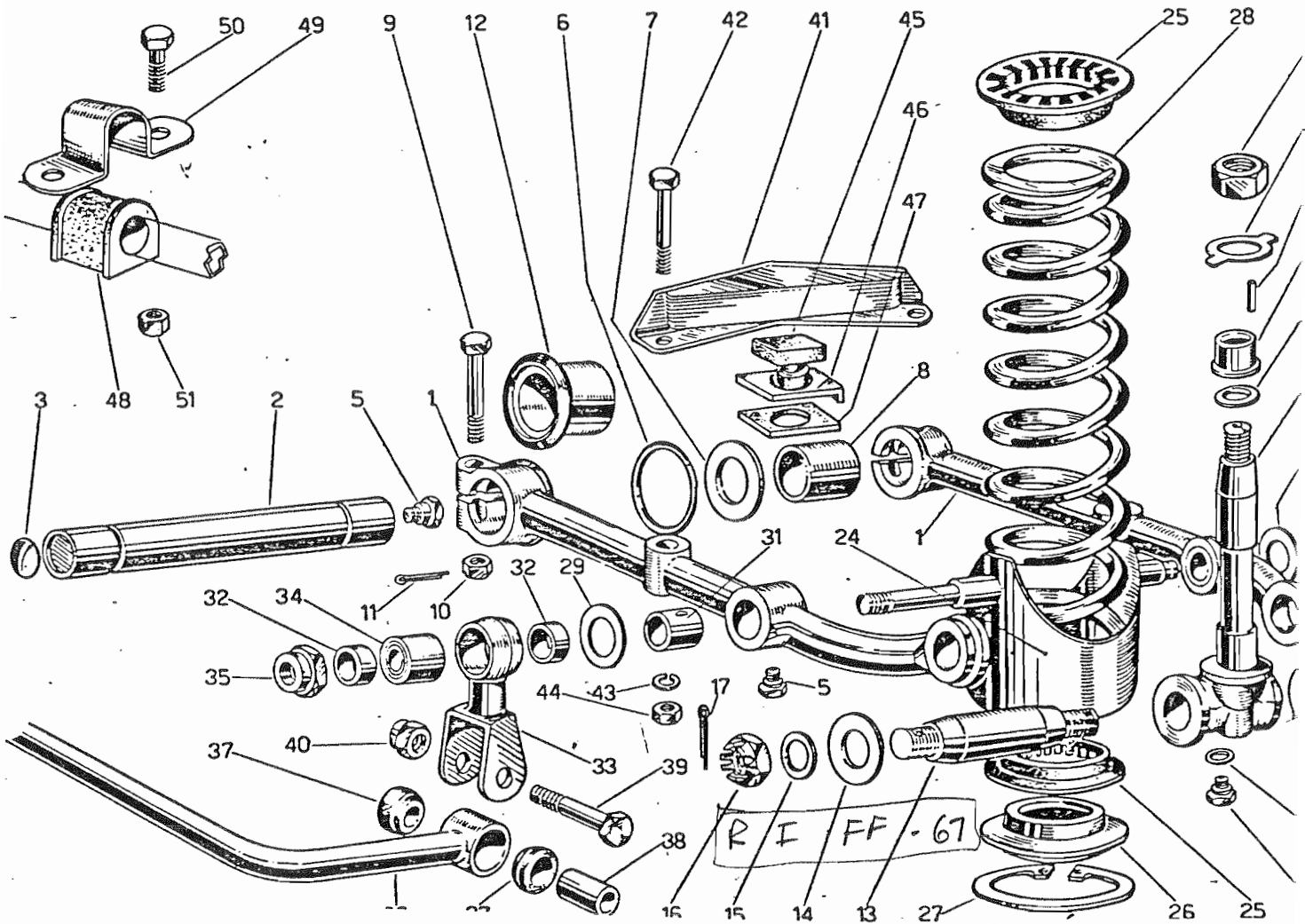
SOSPENSIONE ANTERIORE - BRACCI INFERIORI
