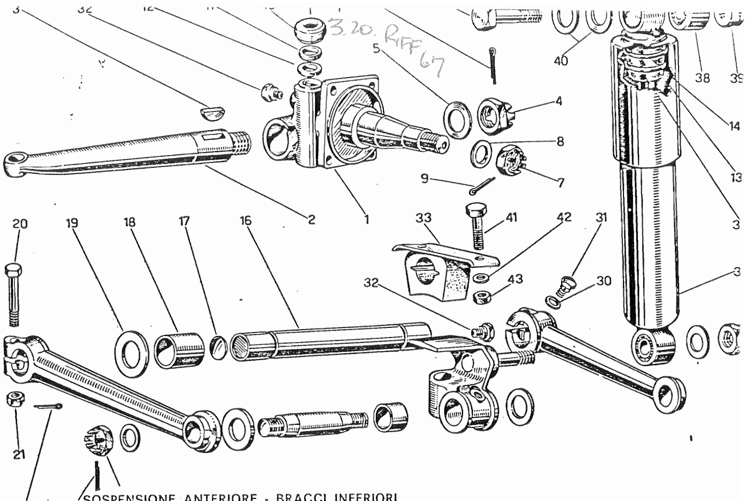
SOSPENSIONE ANTERIORE - BRACCI INFERIORI
