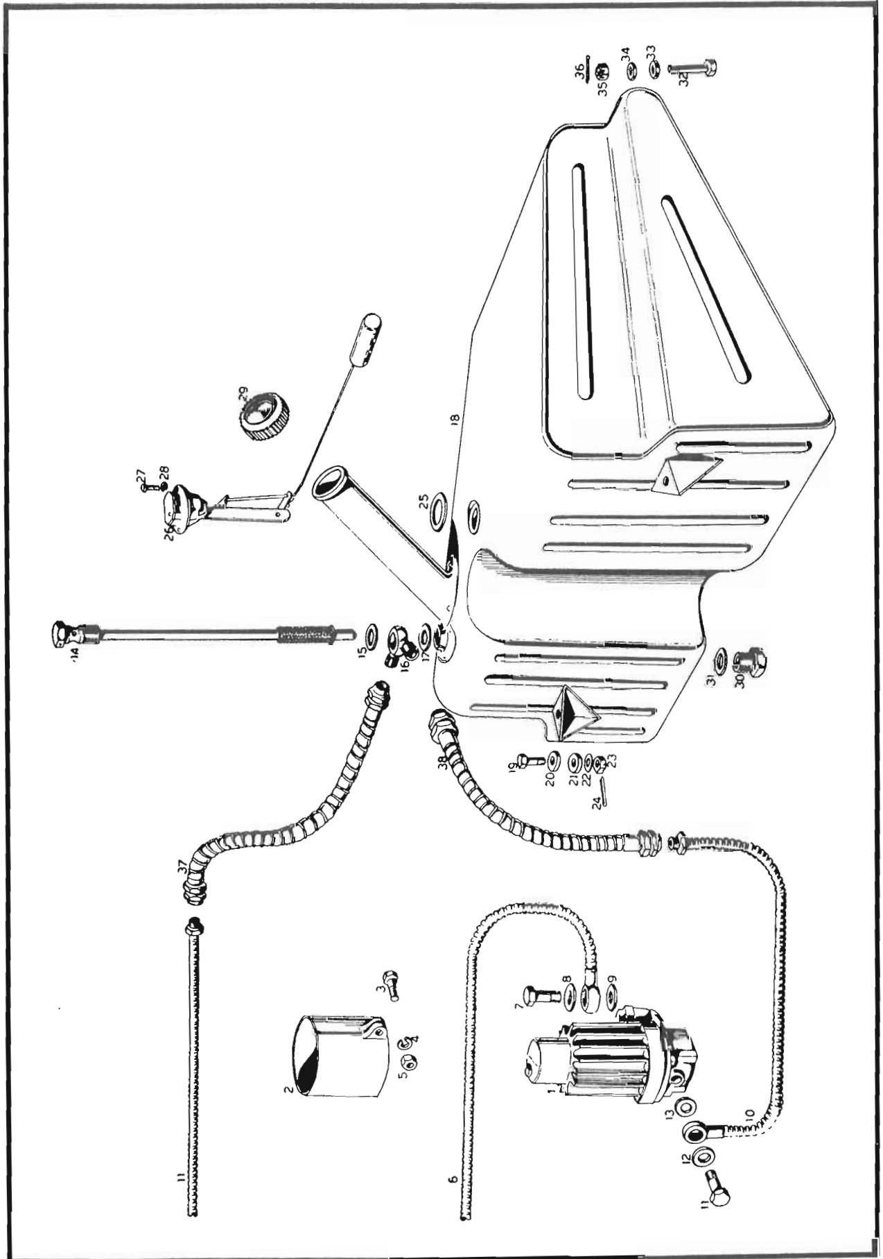
Tavola 10 - Serbatoio carburante con accessori e pompa elettrica
