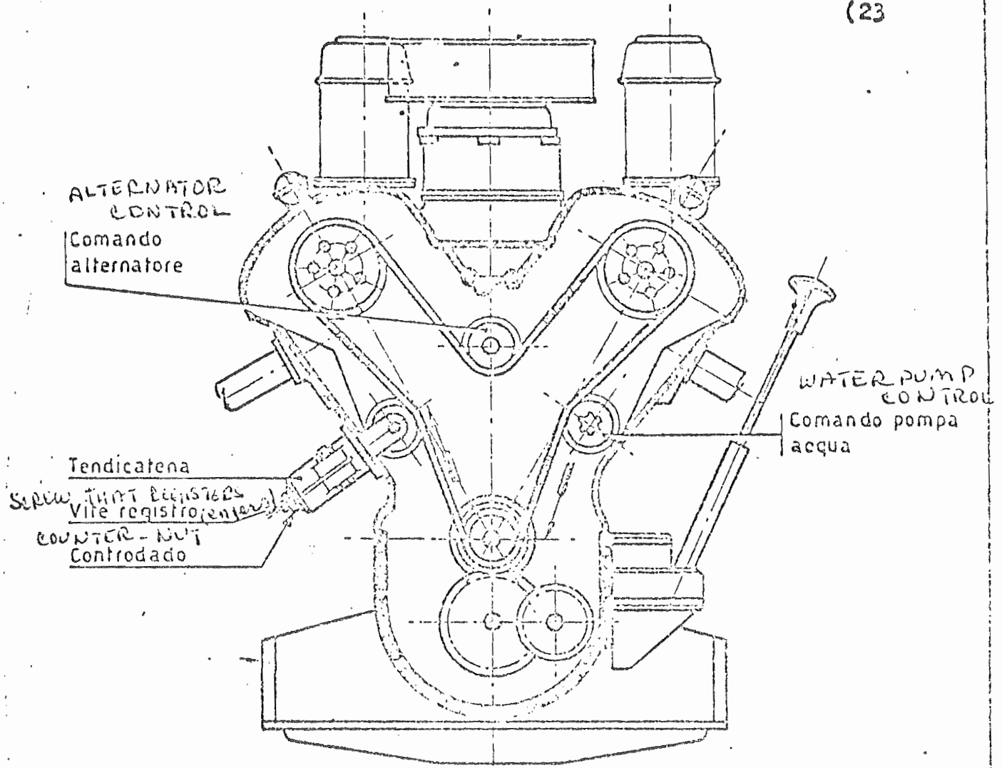
Fig. 3 - CATENA DISTRIBUZIONE (CHAIN DISTRIBUTION)
