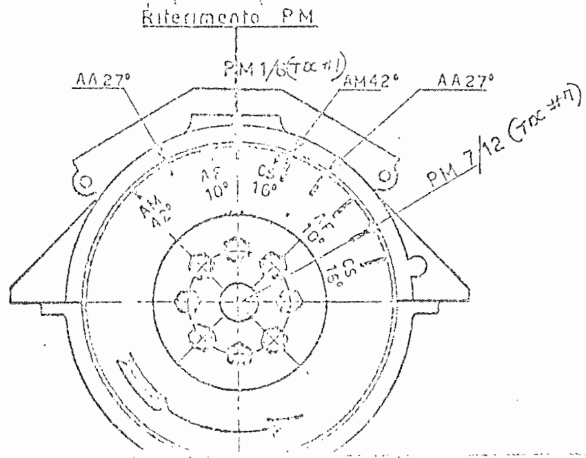
Fig. 3 - CATENA DISTRIBUZIONE (CHAIN DISTRIBUTION)
